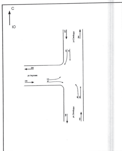
Условные обозначения: 30 - Интенсивность движения, привед. авт. в час ← - Направление движения транспорта 131 - Суммарная интенсивность движения, привед. авт. в час
