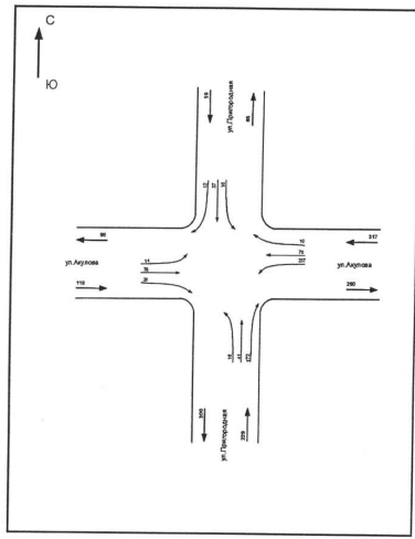
Условные обозначения: 78 - Интенсивность движения, привед. авт. в час ← - Направление движения транспорта 118 - Суммарная интенсивность движения, привед. авт. в час
