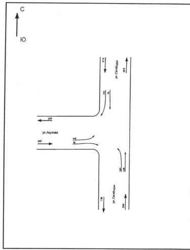
Условные обозначения: 104 - Интенсивность движения, привед. авт. в час ← - Направление движения транспорта 230 - Суммарная интенсивность движения, привед. авт. в час
