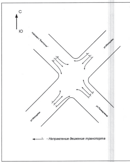
Условные обозначения: 362 - Интенсивность движения, привед. в час; ← - Направление движения транспорта; 362 - Суммарная интенсивность движения, привед. в час
