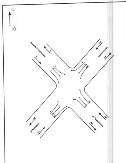
Условные обозначения: 108 - Интенсивность движения, привед. в час; ← - Направление движения транспорта; 312 - Суммарная интенсивность движения, привед. в час
