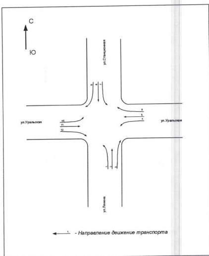
Условные обозначения: 100 - Интенсивность движения, привед. в час; ← - Направление движения транспорта; 251 - Суммарная интенсивность движения, привед. в час
