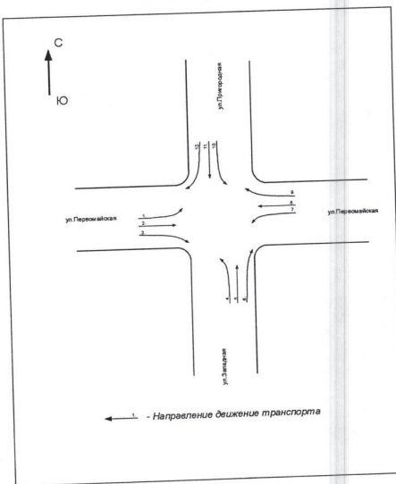
Схема направлений движения на перекрестке улиц Первомайская - Западная (узел А8)
