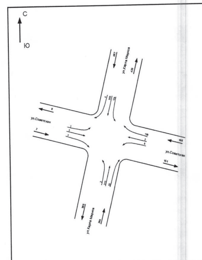
Условные обозначения: 272 - Интенсивность движения, привед. в час; ← - Направление движения транспорта; 294 - Суммарная интенсивность движения, привед. в час
