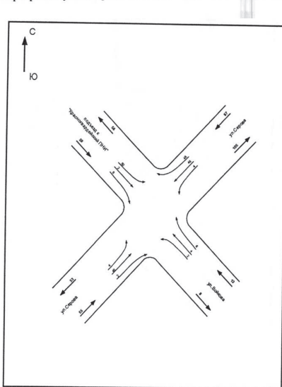
Рисунок 48 – Картограмма распределения интенсивности движения на перекрестке улиц Серова - Войкова в утренний пик (узел К1)
