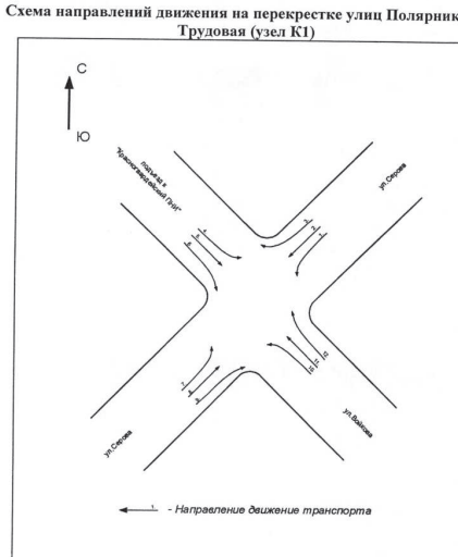
Схема направлений движения на перекрестке улиц Полярников - Трудовая (узел К1)
