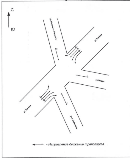
Схема направлений движения на перекрестке улиц Ленина - Новая (узел П)
