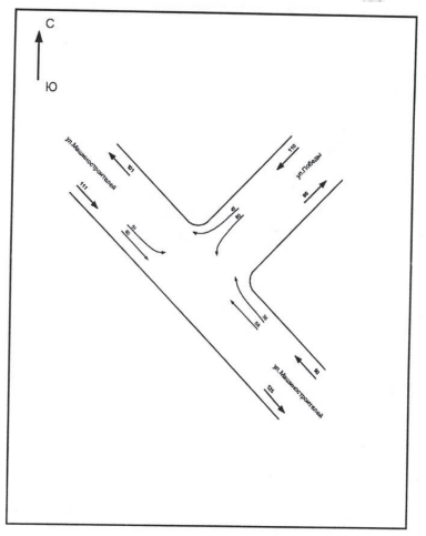
Рисунок 46 – Картограмма распределения интенсивности движение на перекрестке улиц Машиностроителей – Победы в утренний пик (узел Б8)
