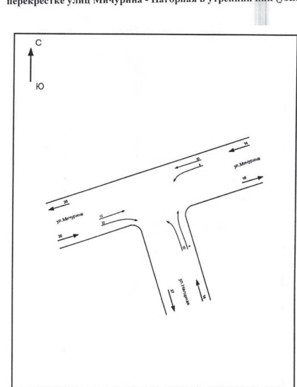
Рисунок 50 – Картограмма распределения интенсивности движения на перекрестке улиц Мичурина - Нагорная в утренний пик (узел К2)
